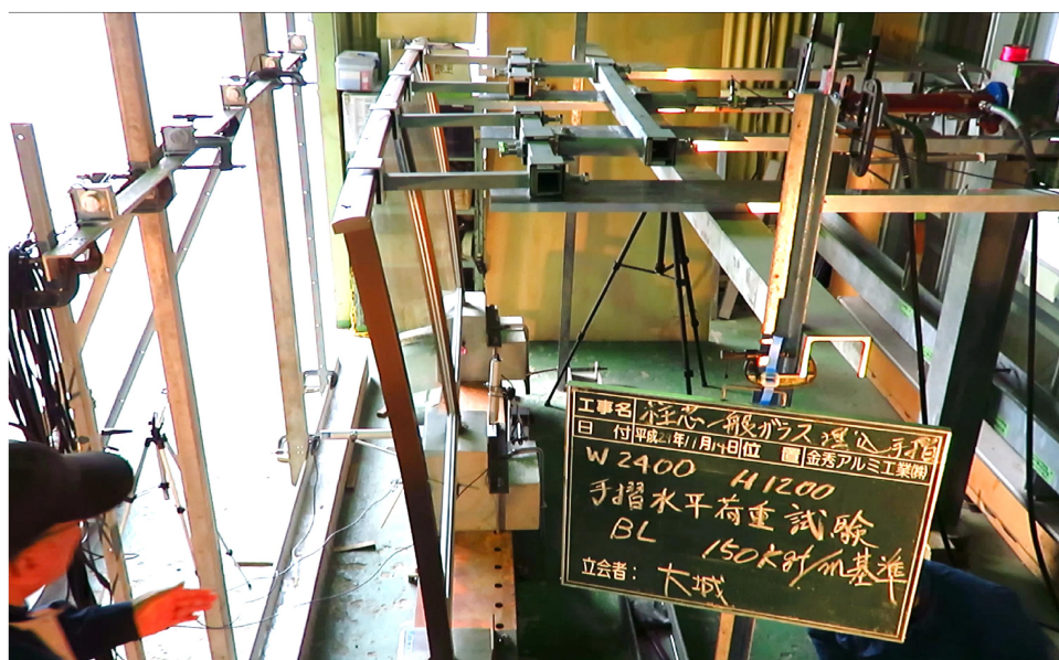
写真2 破壊の状態
